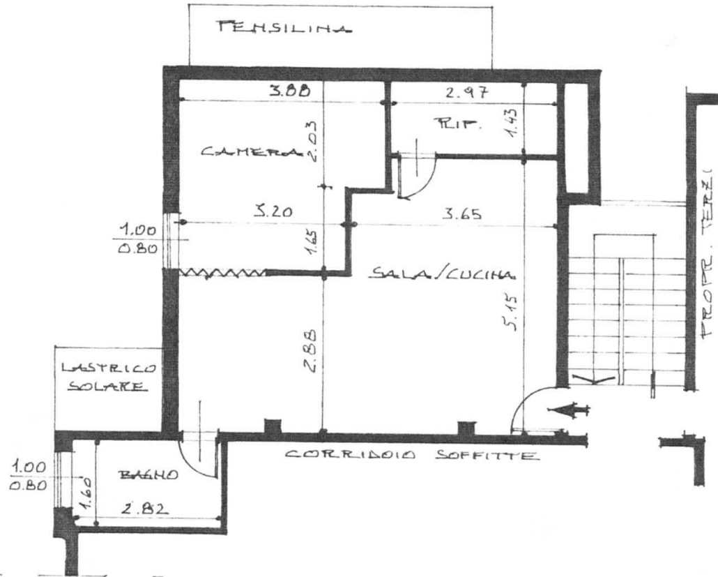
PIANTA PIANO MANSARDATO STATO ATTUALE
